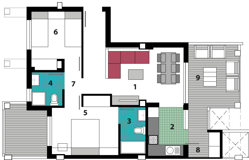
Planta 1°-N°5
