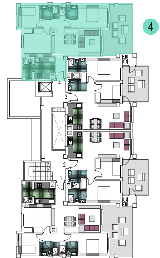
(PLANTA 2º )
