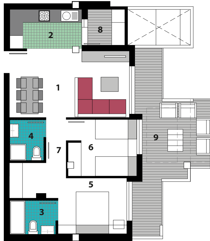
Planta 2°-N°2
