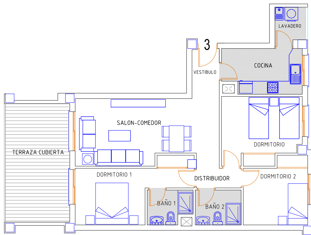
PLANTA 4º - 3
