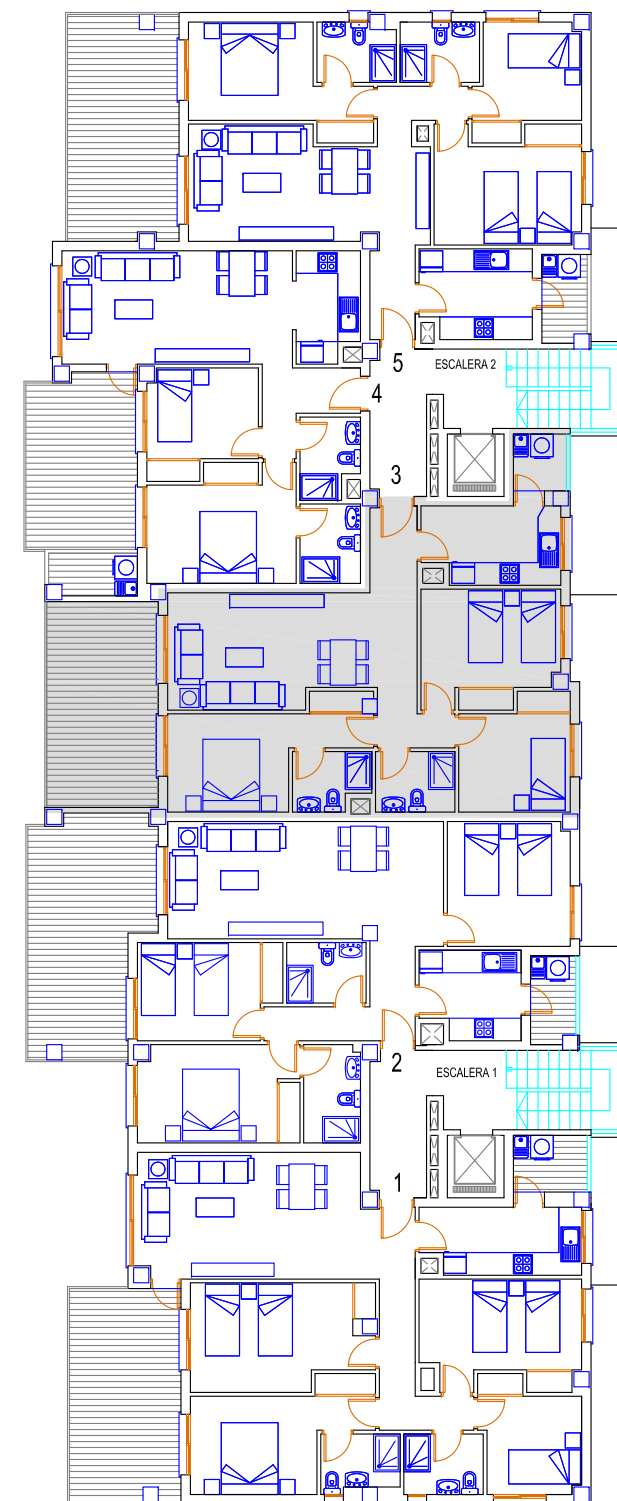
PLANTA 4º
