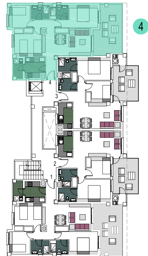
(PLANTA 4º)
